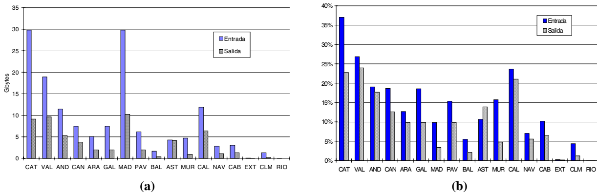
Figura 4. Carga de tráfico por enlace troncal a) Gbytes diarios transmitidos b) utilización media diaria
