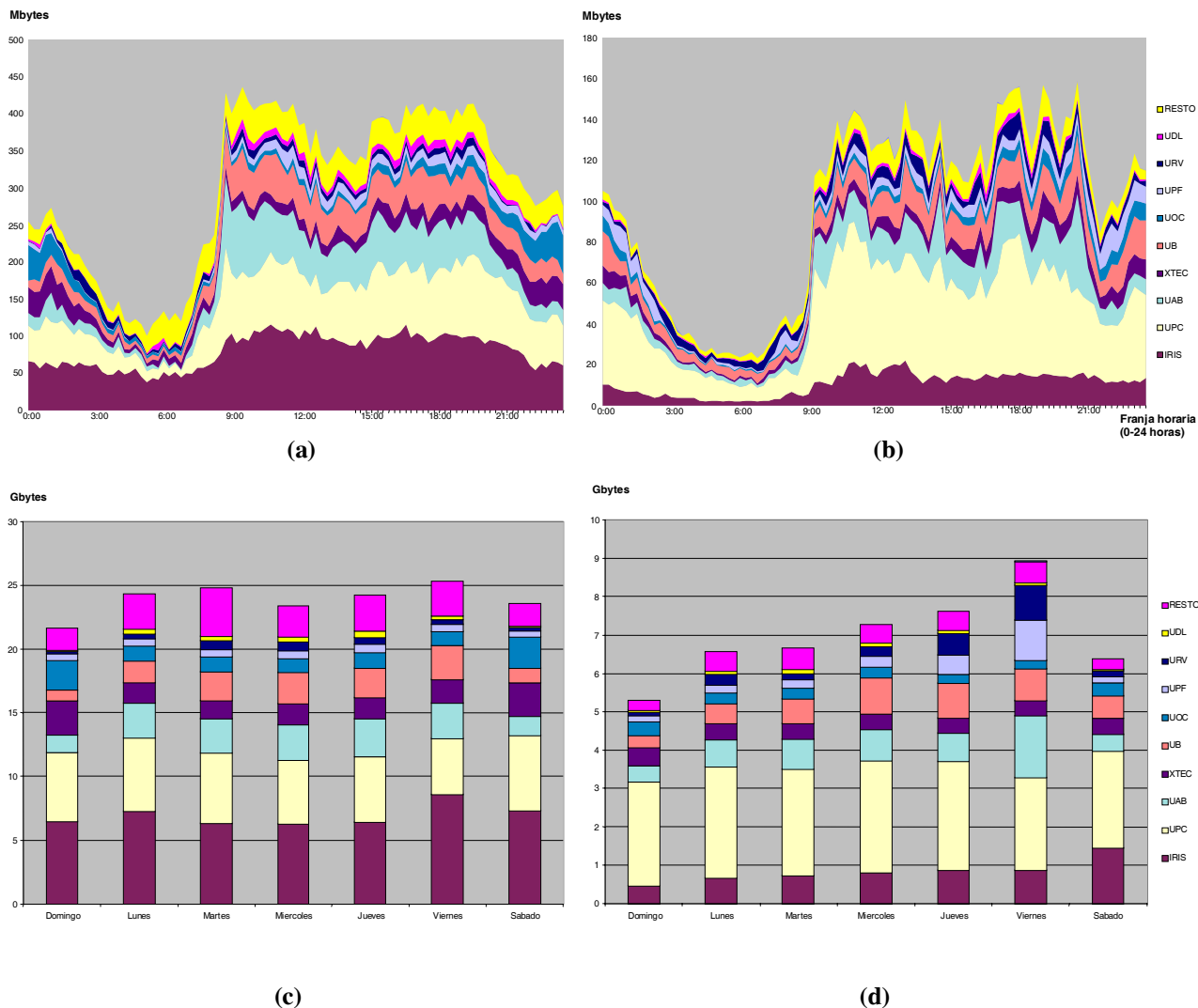
Figura 11. Distribución de tráfico por entidades a) evolución horaria del tráfico de entrada b) evolución horaria del tráfico de salida c) evolución semanal del tráfico de entrada d) evolución semanal del tráfico de salida
