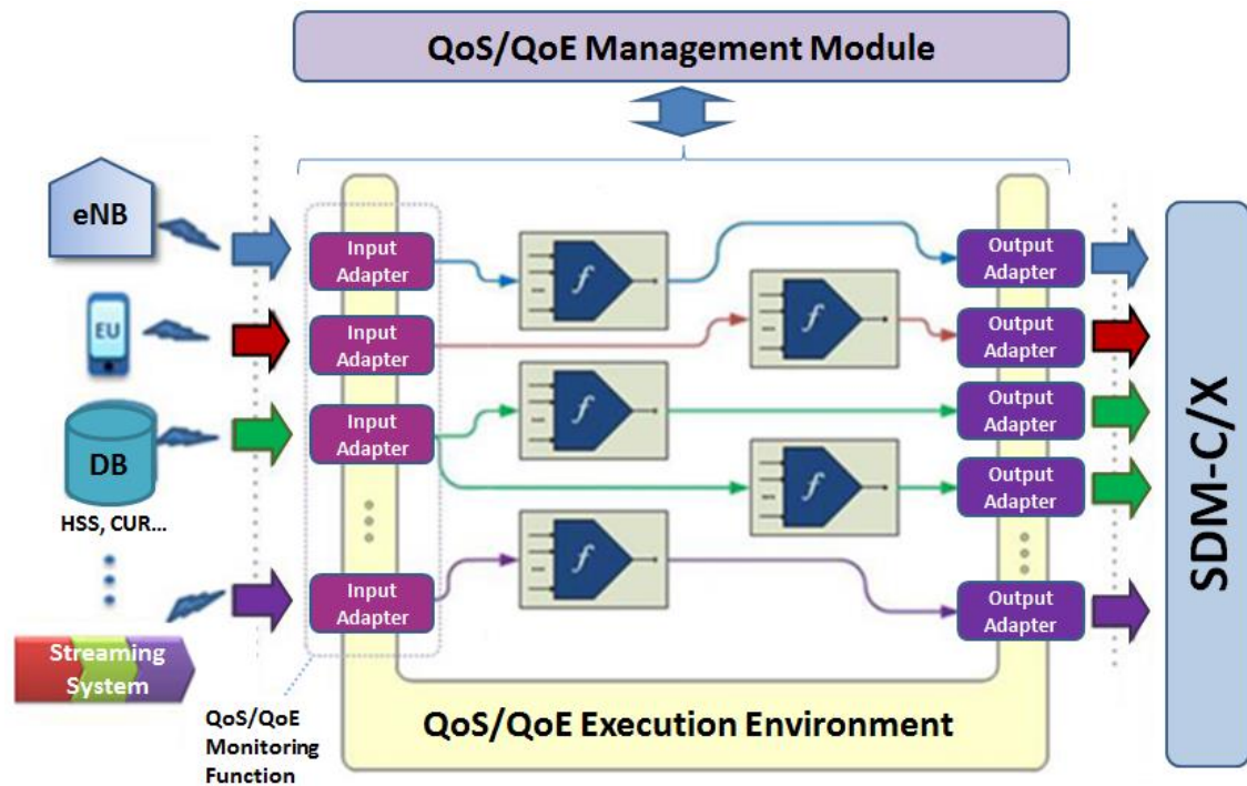
Figure-2-4: 5G NORMA QoE/QoS Framework.
